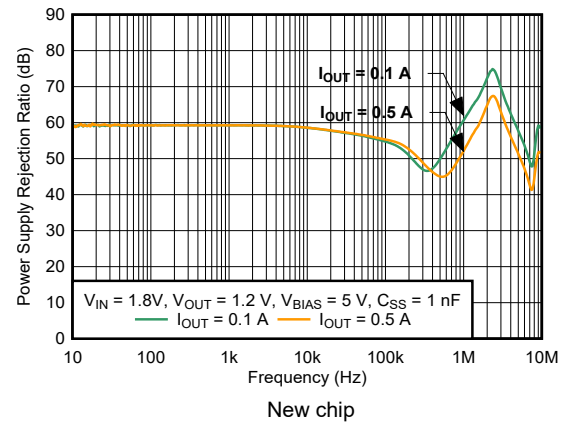
5-14. V_{BIAS} PSRR vs Frequency
