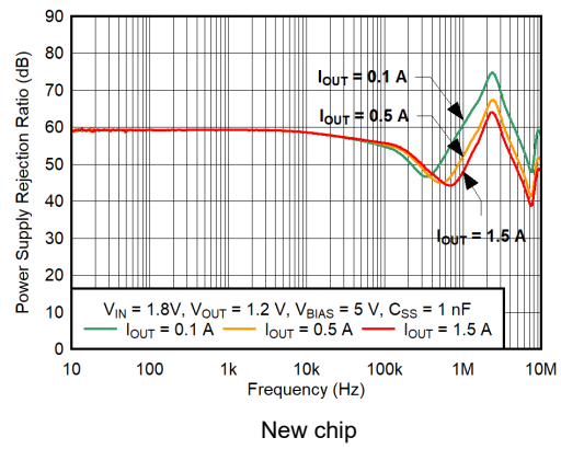
5-16. V_{BIAS} PSRR vs Frequency
