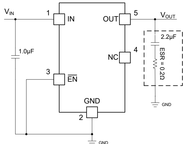
代表的なアプリケーション回路
