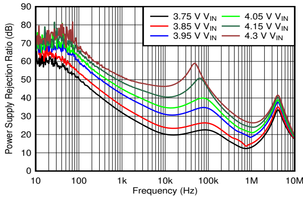
FIG 6-25. PSRR vs V_{IN}
