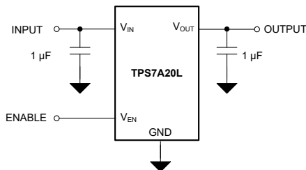
概略回路図
