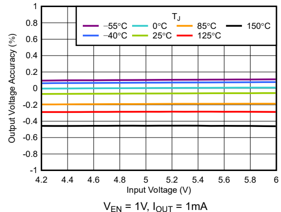
图 5-6. Output Voltage Accuracy vs V_{IN}
