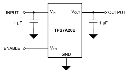
アプリケーション概略回路図
