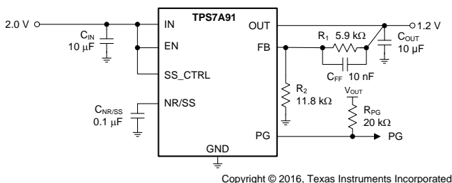
代表的なアプリケーション回路
