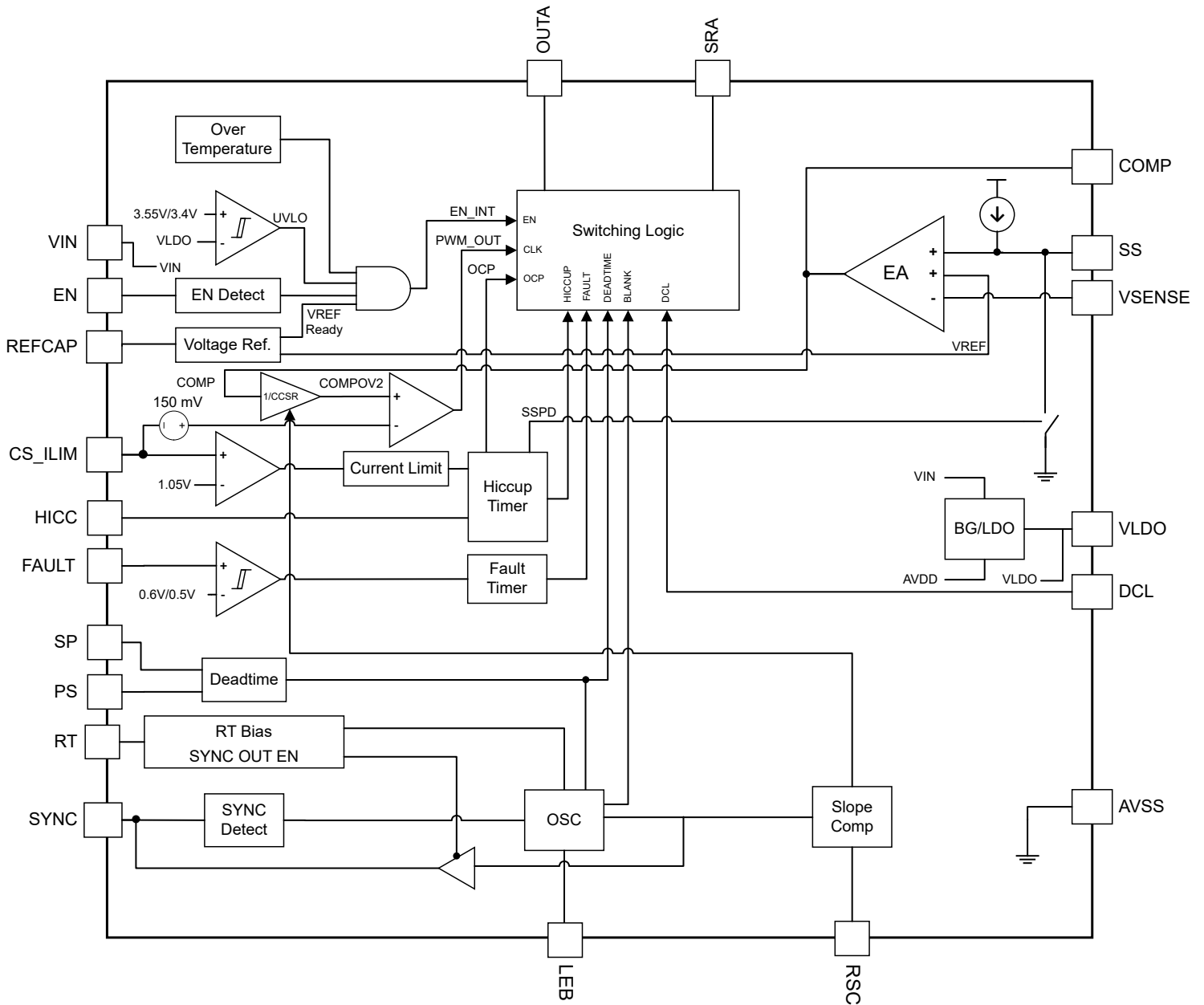
图 9-2. TPS7H5002-SP 功能块图
