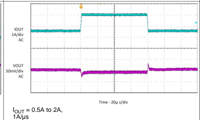
图 27. Load Transient
