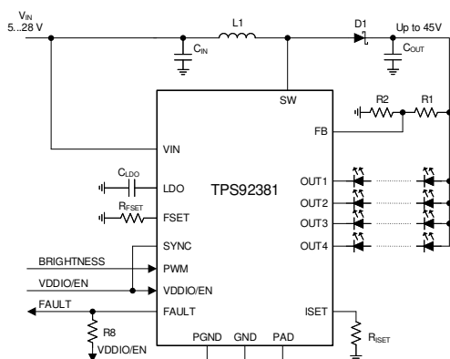
概略回路図
