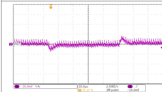
8-4. 5-A Transient Load Step
