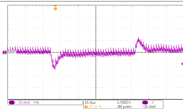
8-5. 10-A Transient Load Step
