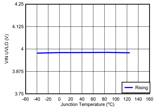
5-8. Vin UVLO
