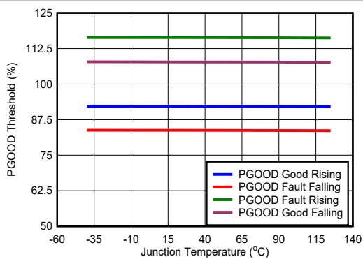
5-9. PG Threshold
