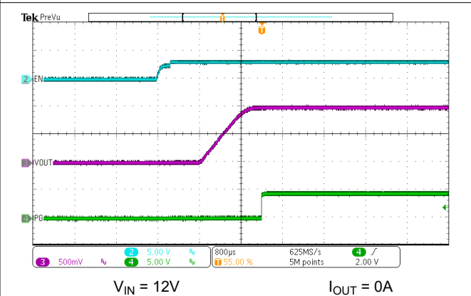
7-9. EN Start-Up – No Load
