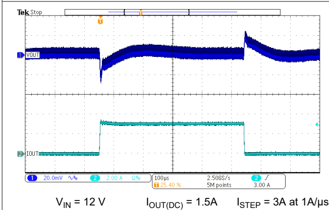
図 7-8. Load Transient
