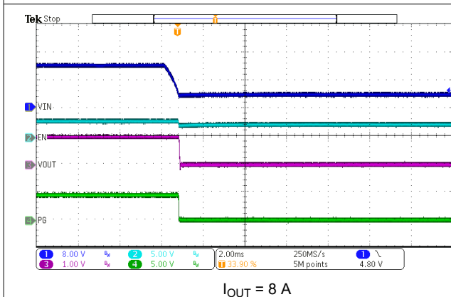
7-14. VIN Shutdown
