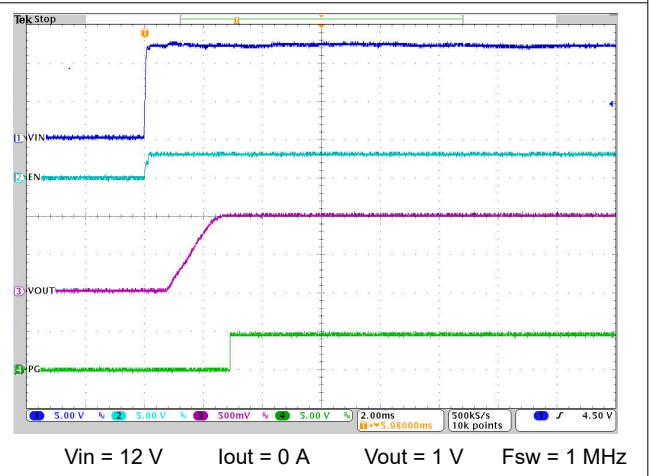
图 8-13. VIN Start-Up
