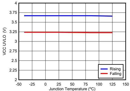
图 6-8. V CC UVLO
