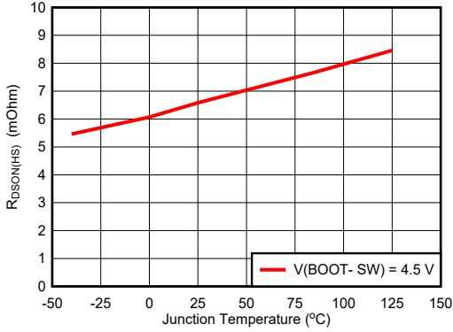
图 6-1. High-Side FET Rd ON
