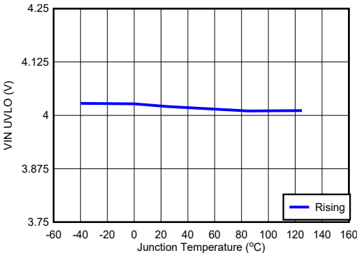
图 6-7. V IN UVLO
