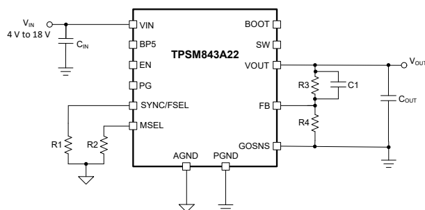
TPSM843A22 のアプリケーション概略図
