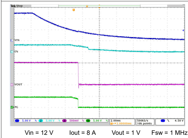
图 8-14. VIN Shutdown
