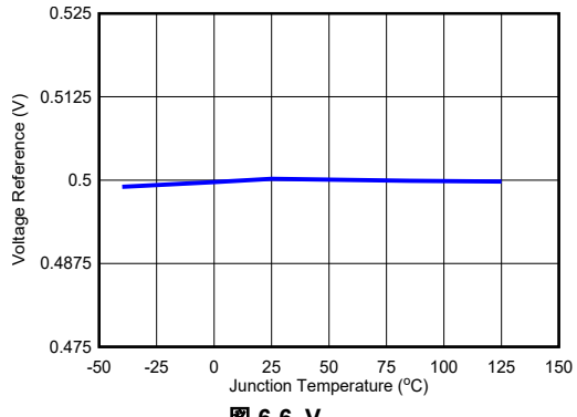
图 6-6. V REF
