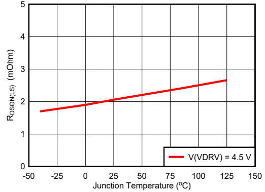
图 6-2. Low-Side FET Rd ON
