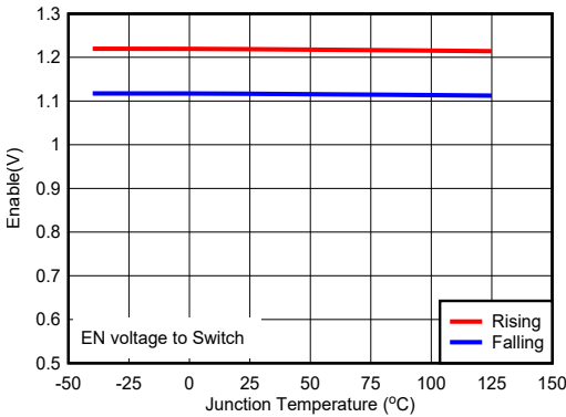
图 6-5. Enable Voltage
