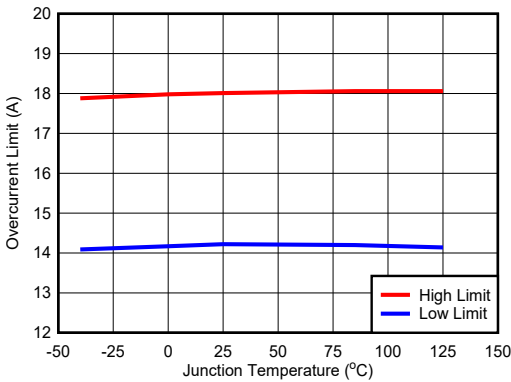
图 6-3. Overcurrent Limit
