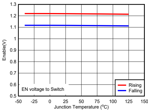
6-5. Enable Voltage
