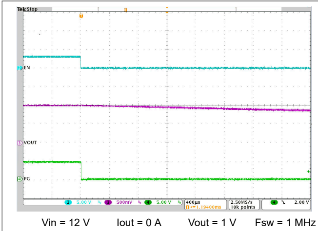
8-10. EN Shutdown
