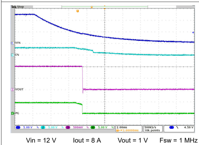
8-14. VIN Shutdown
