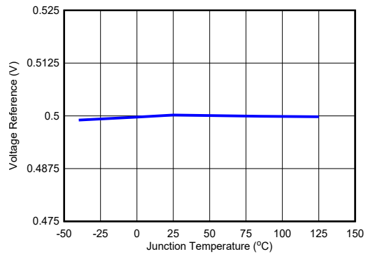
6-6. V REF
