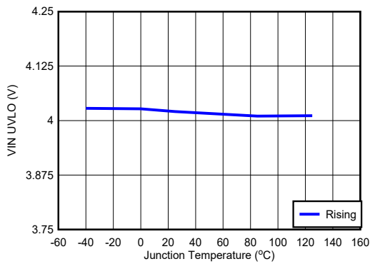
Figure 6-7. VIN UVLO
