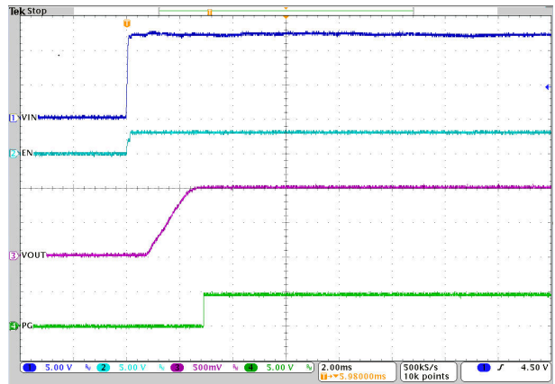
图 8-11. EN Start-Up – With Load
