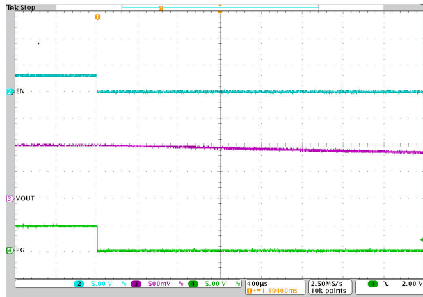
图 8-10. EN Shutdown
