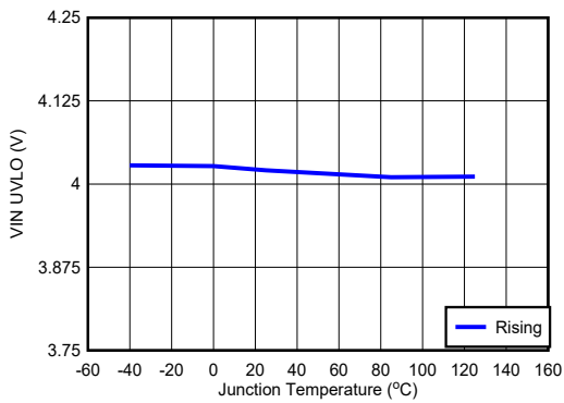
图 6-7. V_{IN} UVLO
