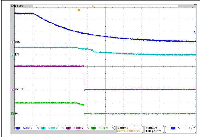
☒ 8-14. VIN Shutdown
