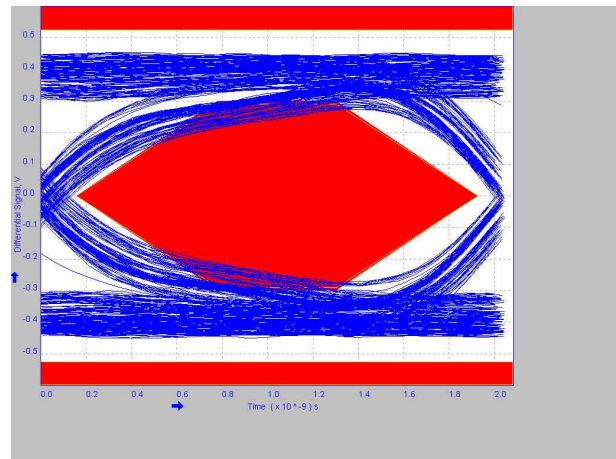
9-8. 5 Meter Without TUSB217A
