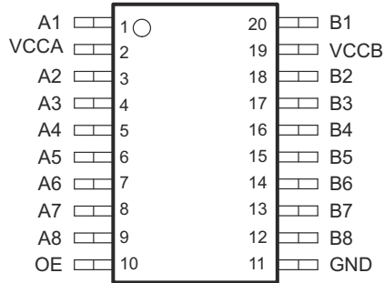
図 4-3. PW パッケージ、20 ピン TSSOP (上面図)
