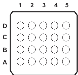
図 4-1. ZXY パッケージ、20 バンプ (底面図)
