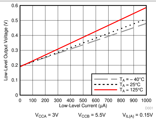
図 5-2. Low レベル出力電圧 ( V_{OL(Bx)} ) と Low レベル電流 ( I_{OL(Bx)} ) との関係
