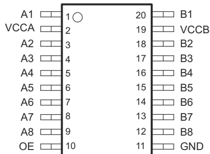
図 4-1. PW パッケージ、20 ピン TSSOP (上面図)
