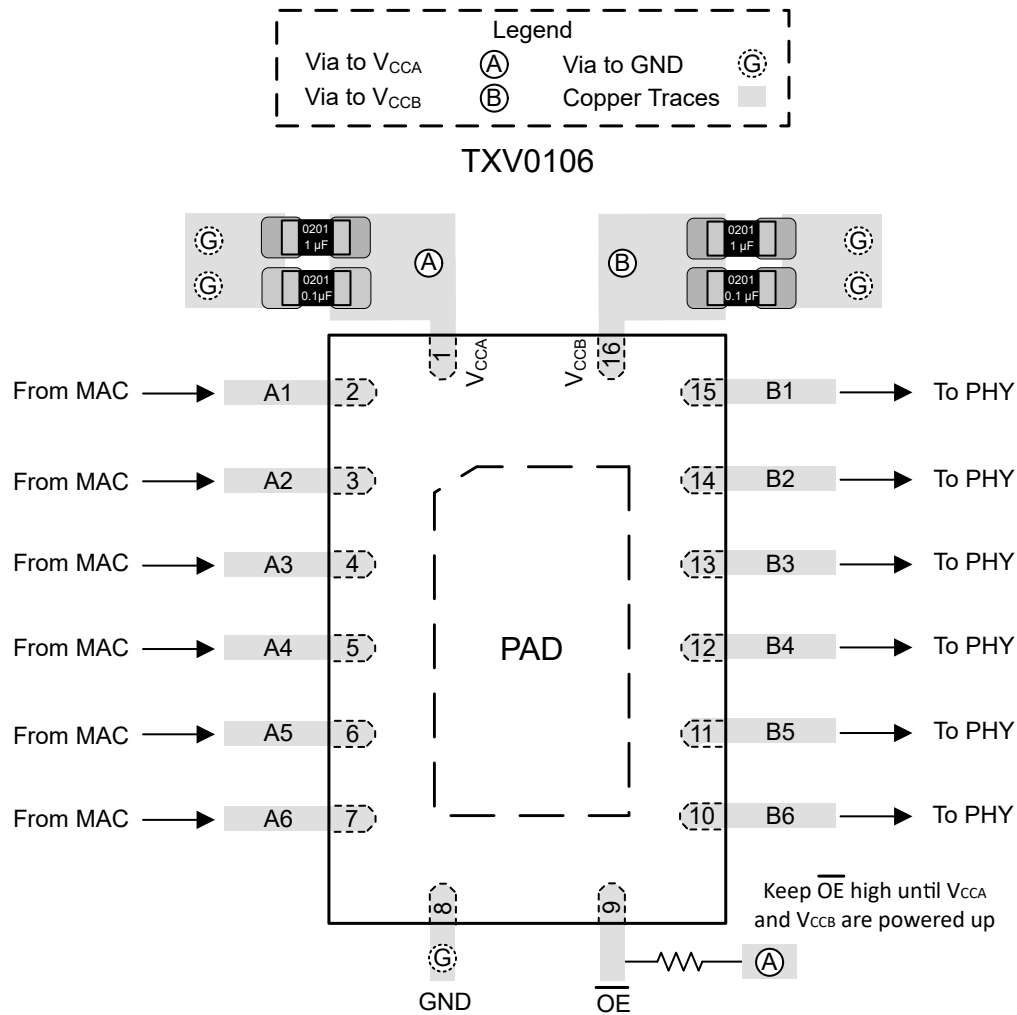
図 8-6. レイアウト例 – TXV0106
