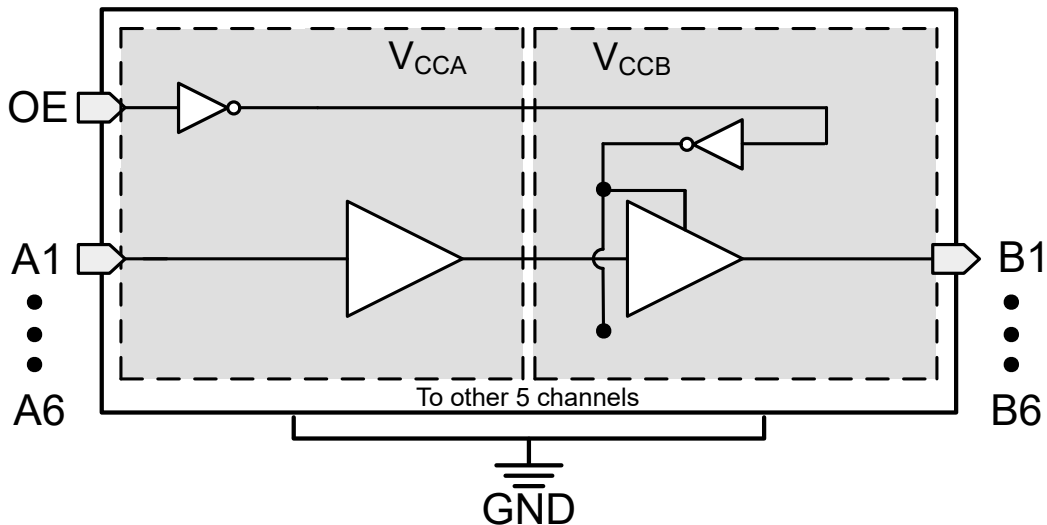
図 7-1. TXV0106 の機能ブロック図
