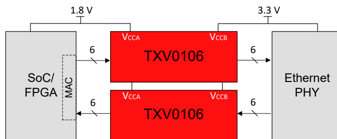
RGMII アプリケーションの TXV0106
