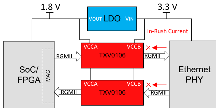
図 8-5. 電源の絶縁に TXV0106 を使用
