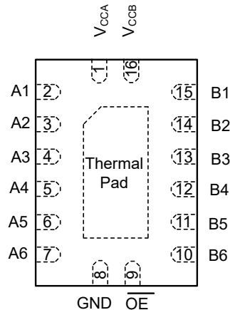
図 4-1. BQB パッケージ、16 ピン WQFN (上面図)
