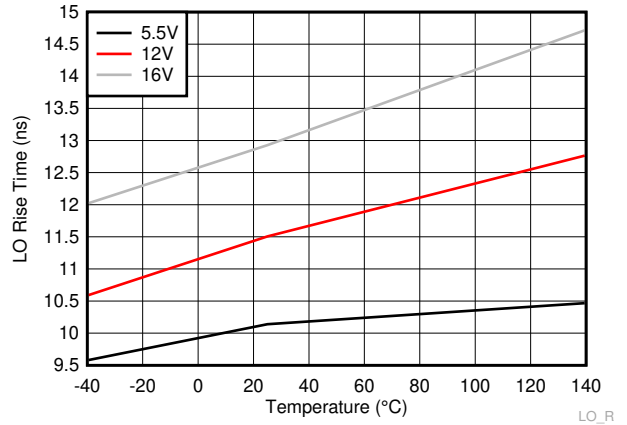
6-22. LO Rise Time
