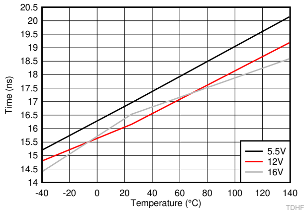
6-27. HO Rise andamp; Fall Time
