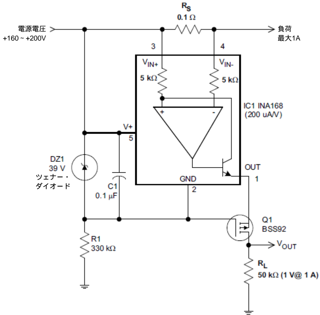
図1 INA168の電圧範囲を拡張する回路の例
