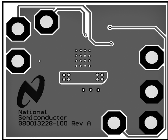
Bottom Layer
