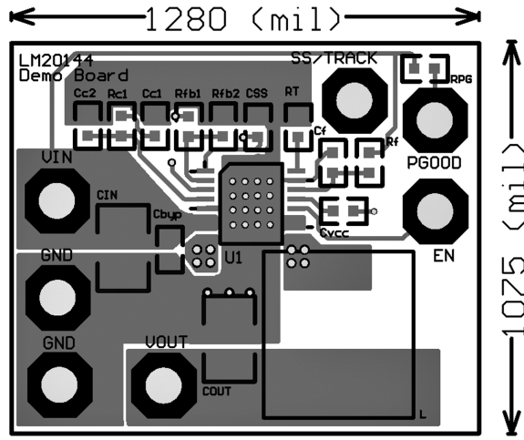
Top Layer
