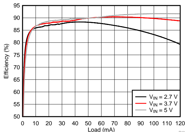
バックライト効率、4P6S
