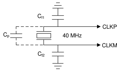
图 8-4. Crystal Implementation
