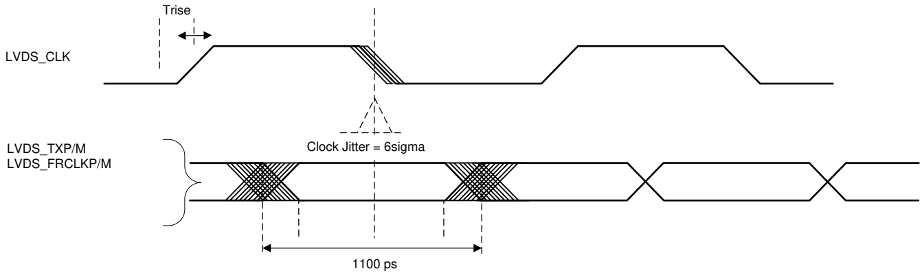
図 8-13. Timing Parameters
