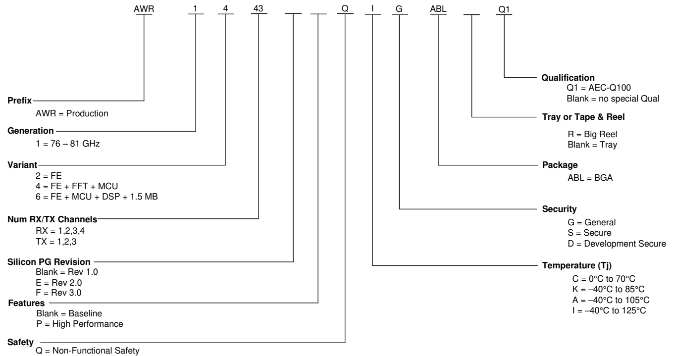
図 11-1. Device Nomenclature
