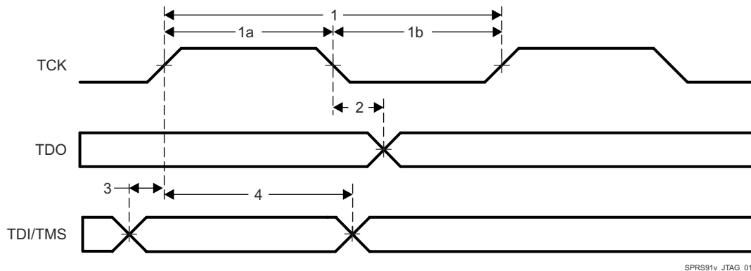
図 8-17. JTAG Timing
