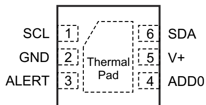
図 5-1. DRV パッケージ 6 ピン WSON 上面図
