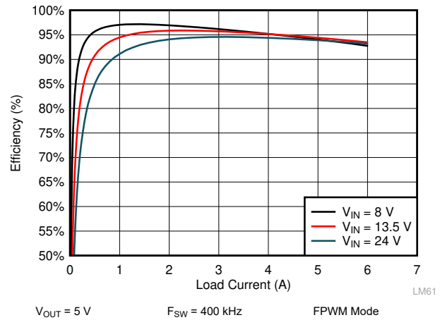
图 10-10. LM61460-Q1 Efficiency
