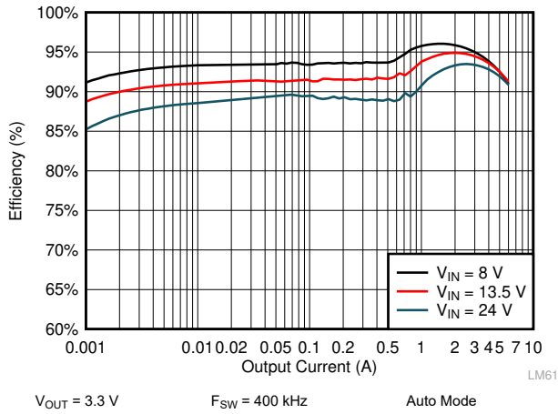
图 10-5. LM61460-Q1 Efficiency
