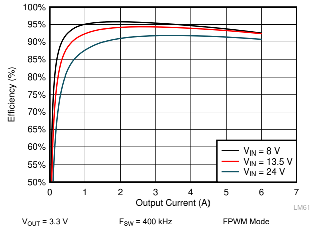
图 10-6. LM61460-Q1 Efficiency
