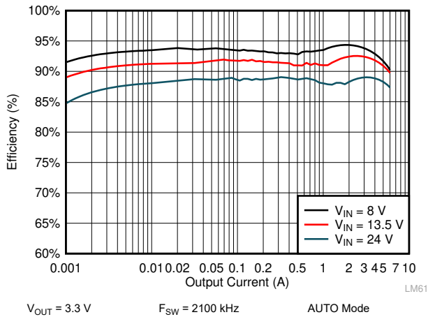
图 10-7. LM61460-Q1 Efficiency
