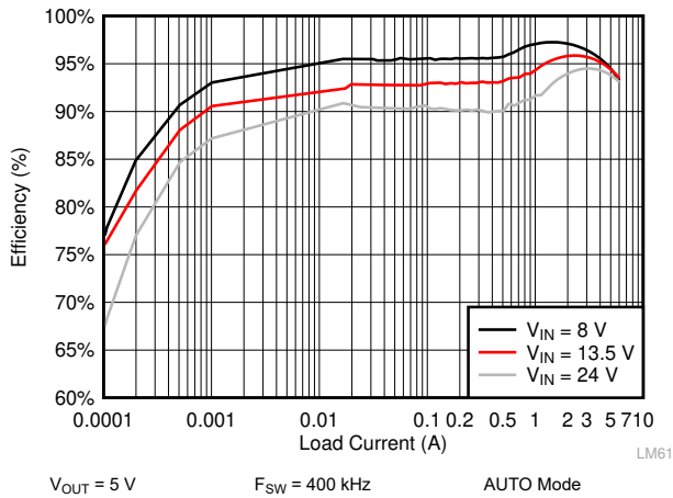
图 10-9. LM61460-Q1 Efficiency
