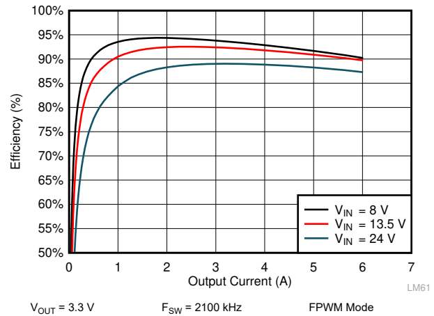
图 10-8. LM61460-Q1 Efficiency
