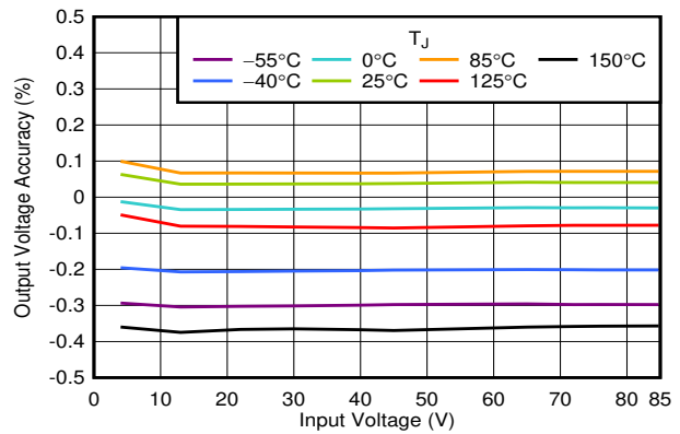
图 6-2. V_{OUT} Accuracy vs V_{IN}
