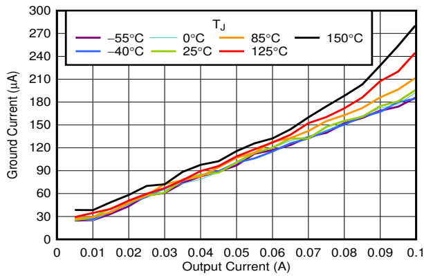
6-7. I_{\text{GND}} vs I_{\text{OUT}}
