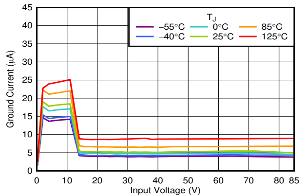
6-8. I_{\text{GND}} vs V_{\text{IN}}
