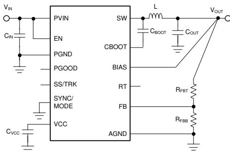
概略回路図
