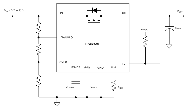
簡略回路図
