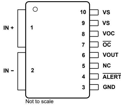
图 5-1. DVG Package 10-Pin SOIC Top View
