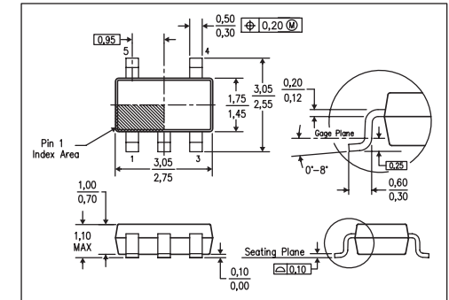
TSOT-23(DCC)パッケージ
