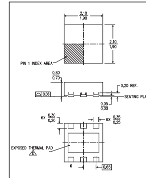
SON パッケージ
