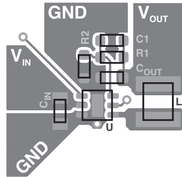
可変電圧製品のレイアウト
