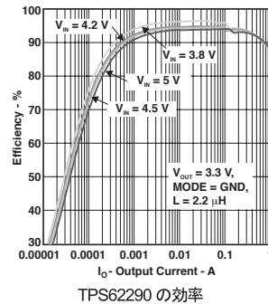
TPS62290 の効率
