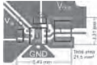
固定電圧製品のレイアウト
