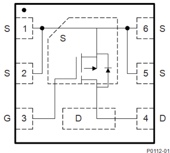
図 22. CSD25310Q2 Device Configuration
