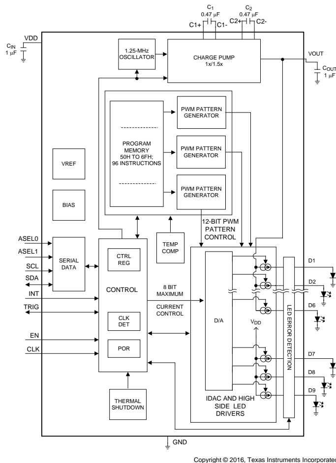
図 21. LP55231 Block Diagram
