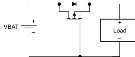
図 3. PMOS FET Power Path
