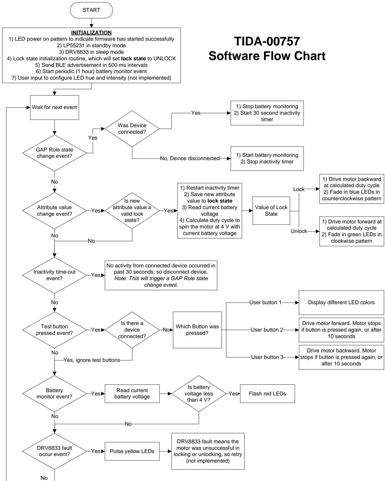
図 16. Software Flow Chart
