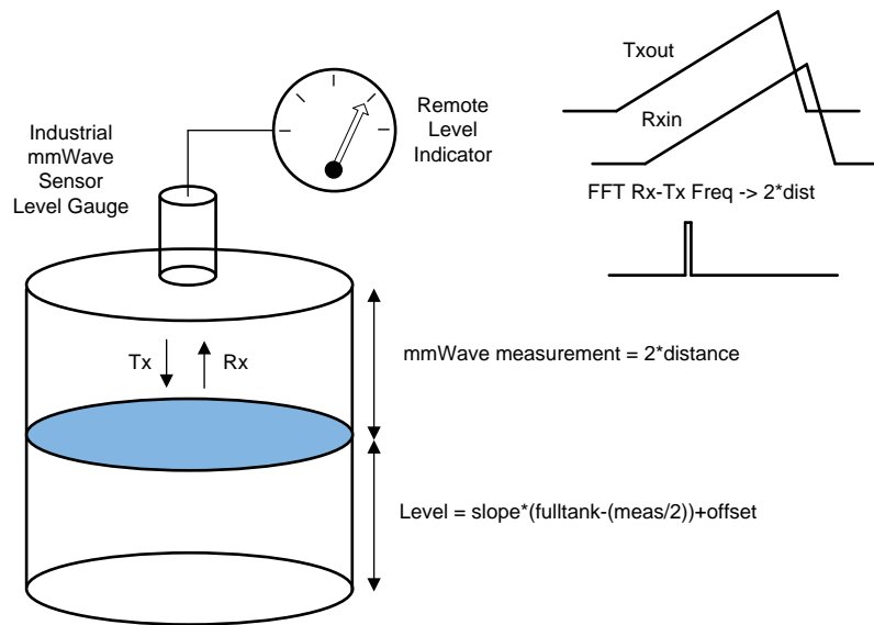
図 1. TIDEP-0091 System Block Diagram
