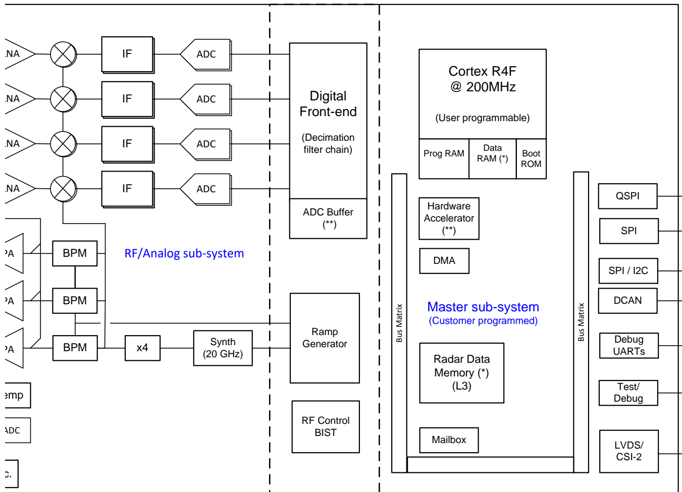
図 5. TIDEP-0091 IWR 1443 mmWave Sensor Block Diagram
