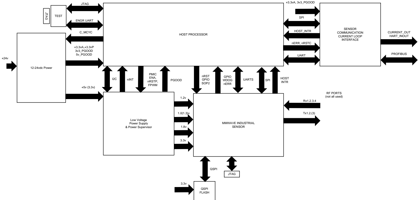
図 2. TIDEP-0091 Block Diagram
