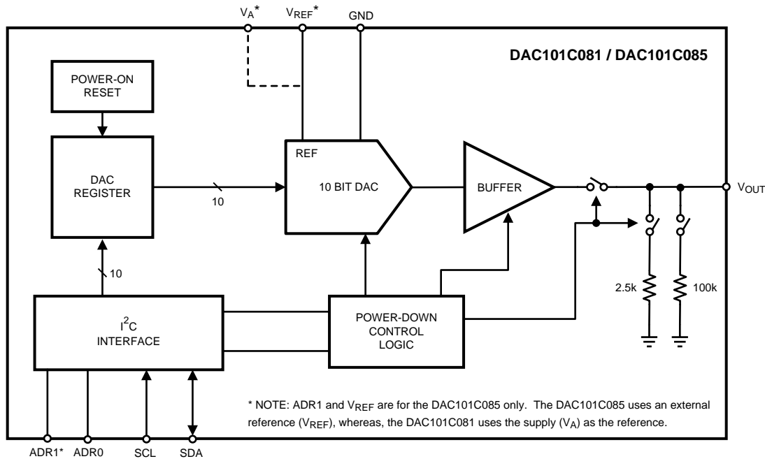
図 4. DAC101C081Q Block Diagram
