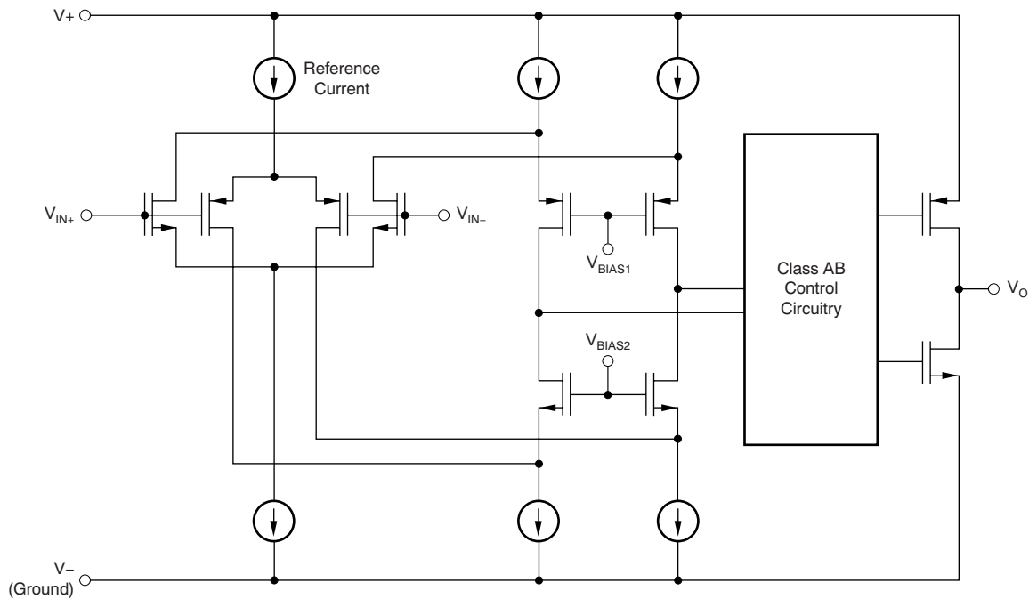
図 5. TLV316-Q1 Block Diagram
