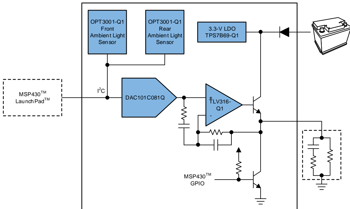
図 1. TIDA-01359 Block Diagram
