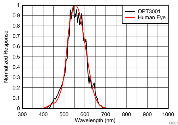
図 3. OPT3001-Q1 Spectral Response
