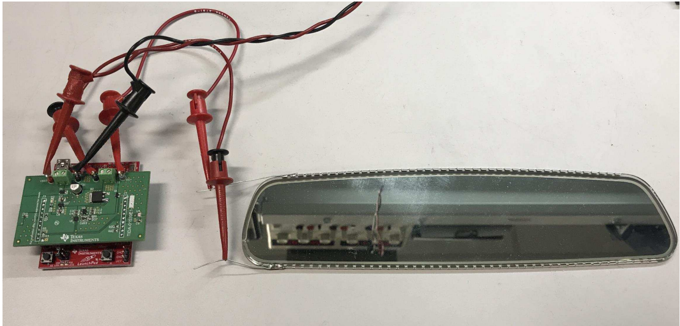
図 14. TIDA-01539 Test Setup
