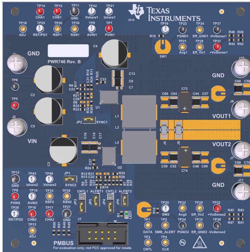
Figure 8-1. TPS546C20AEM2-746 EVM 3D (Top View)
