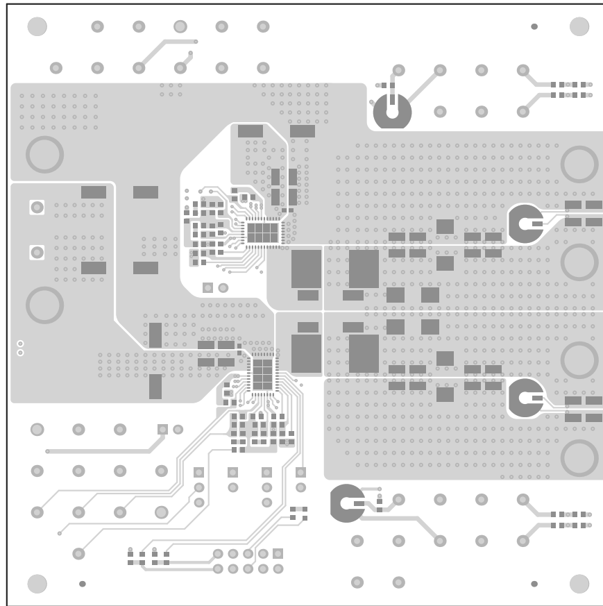
Figure 8-4. TPS546C20AEVM2-746 EVM Top Copper (Top View)
