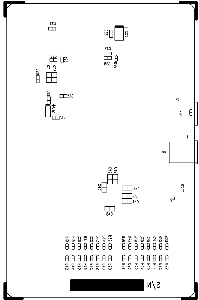
C-6. Bottom Silkscreen
