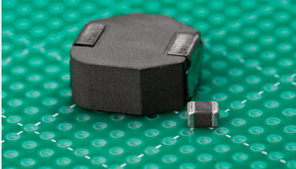
그림 1. 8.2μH 인덕터(400kHz)와 소형 3.3μH 인덕터(2.1MHz)의 크기 비교
