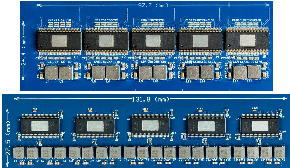
그림 2. 5개의 TAS6754-Q1 클래스 D 증폭기로 구성된 20채널 차량용 오디오 시스템 설계와 TI의 TAS6424E-Q1 클래스 D 증폭기 비교
