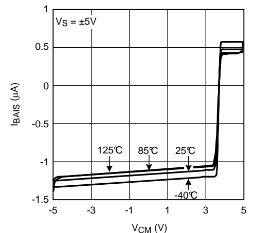
Figure 24. I_{BIAS} vs. V_{CM}
