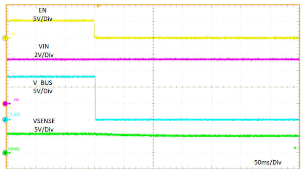
EN = 5 \text{ V to } 0 \text{ V} CC1 = R_d I_{BUS} = 3 \text{ A}
