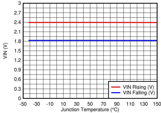
Figure 5-7. VIN UVLO
