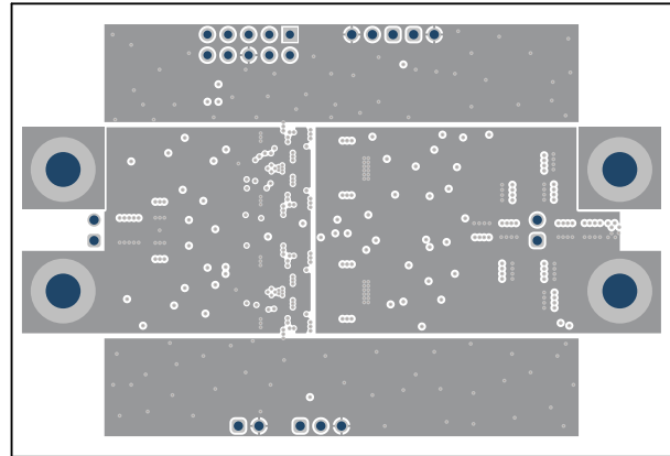
Figure 5-4. Layer 3
