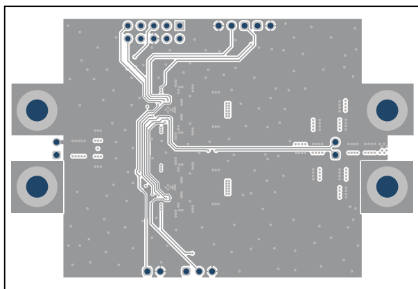
Figure 5-7. Layer 6
