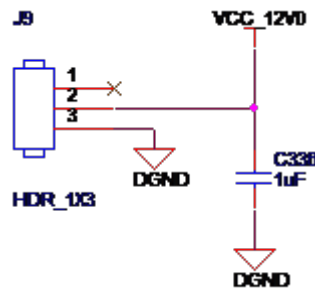
Figure 28. Cooling FAN Header
