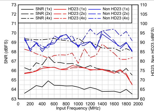
A_{IN} = -4\text{ dBFS} , Dither = EN
