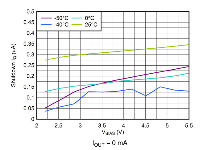
Figure 6-8. V_{\text{BIAS}} Shutdown I_{\text{Q}} vs V_{\text{BIAS}}
