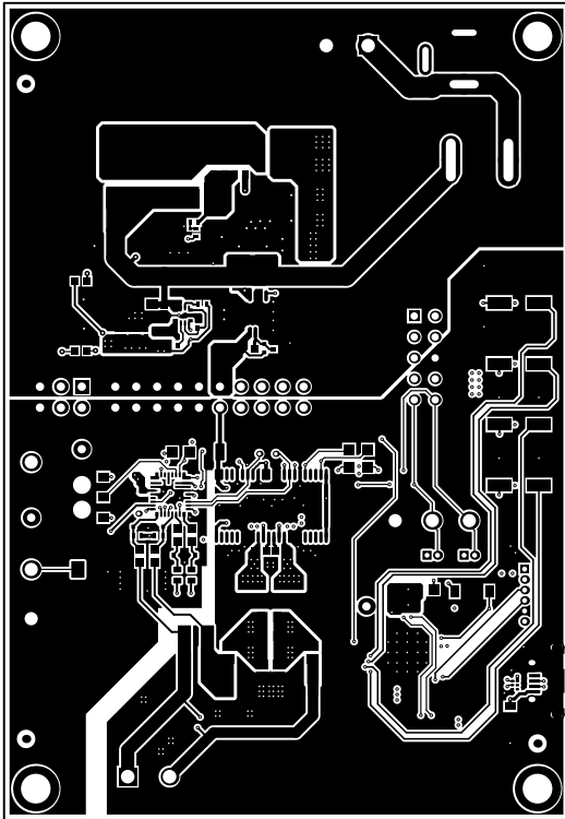
Figure 6-4. Top Layer
