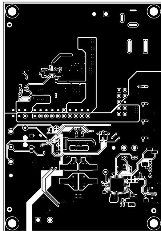
Figure 6-7. Bottom Layer
